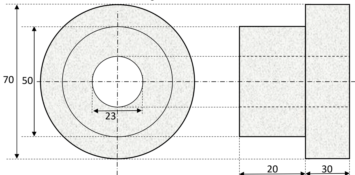
Bague centreur en PET - côtes en mm
