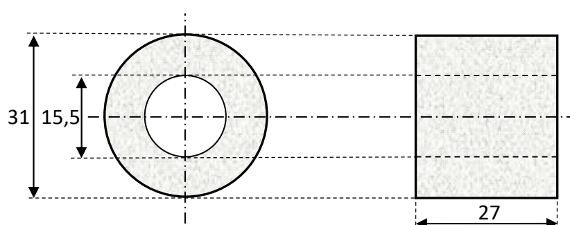
Manchon d'usure en PET durci - côtes en mm
