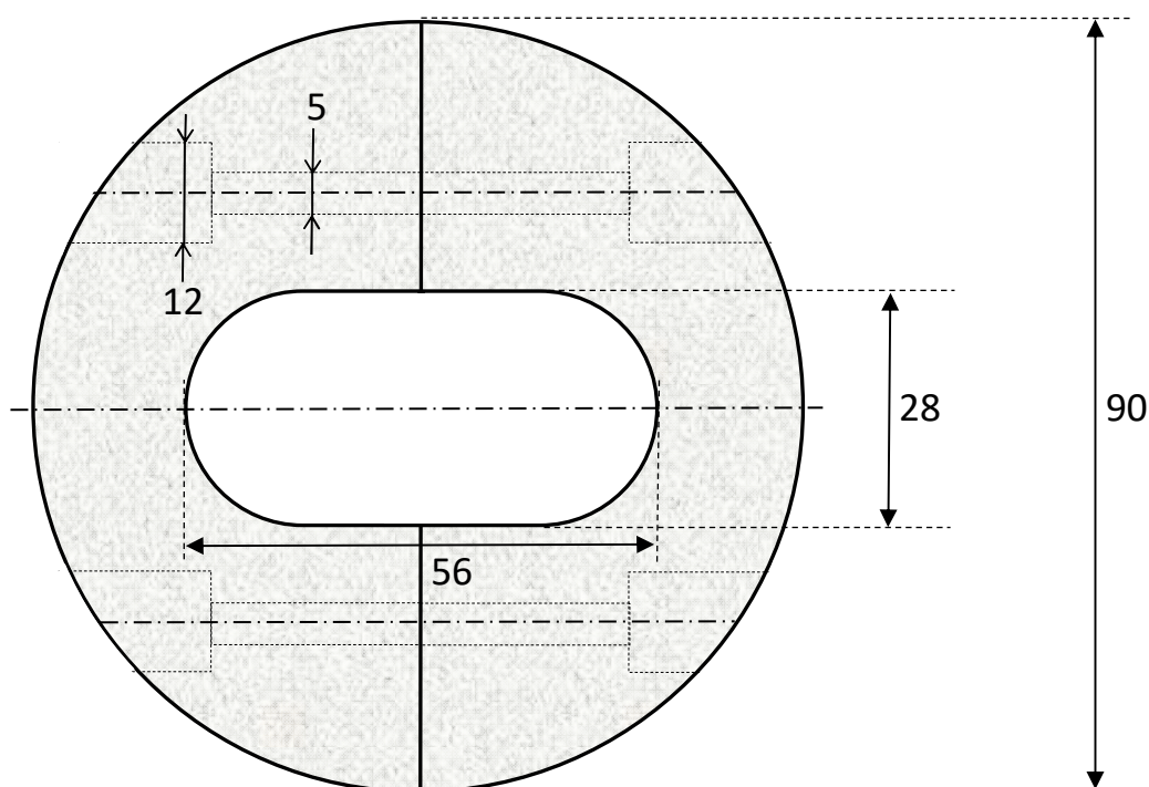
Manchon d'usure en PET durci - côtes en mm
