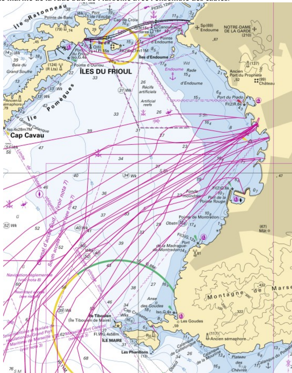
1-carte marine de la rade Sud de Marseille avec l'ensemble des câbles.
