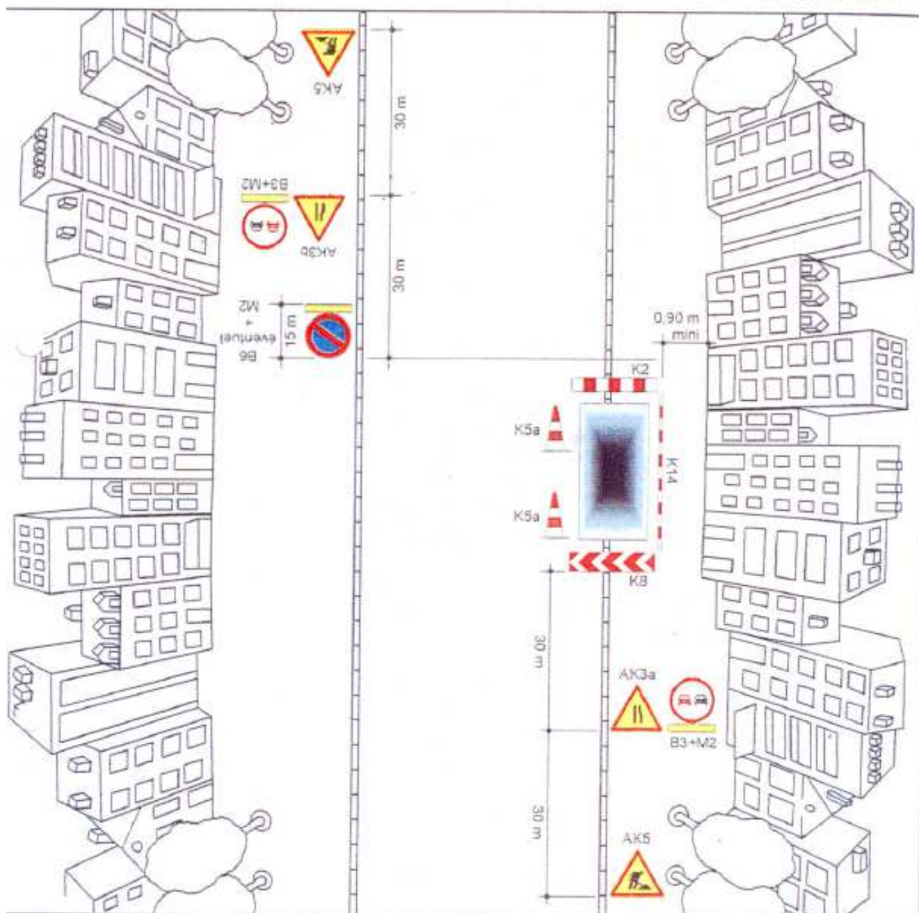
schéma U-13
